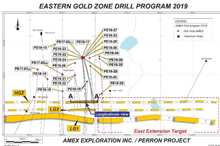
Figure 1: Carte du plan des emplacements des trous forés.
